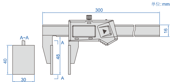
测量钢丝绳直径
